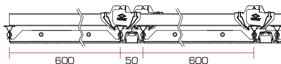
ŘEZ STANDARDNÍ KAZETOU SE ZKOSENÝM OKRAJEM BEVELLED EDGE TILE'S SECTION
