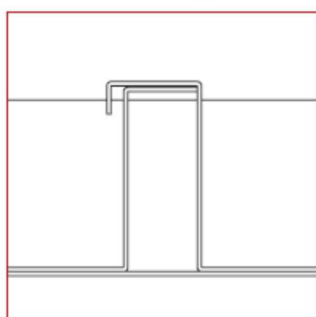
DETAIL ŘEZU SECTION DETAIL
